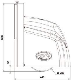
MEDIDA EN MILÍMETROS
